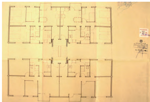
Avantprojecte d'habitatge tipus primera fase, 1961. (Arxiu Municipal de Manlleu)
