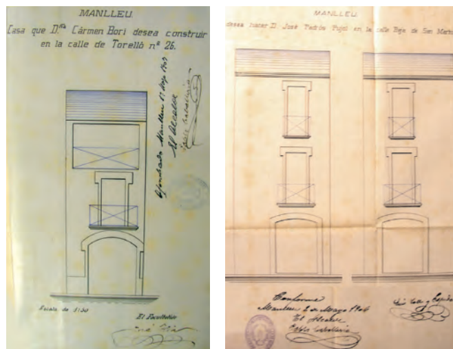
Llicències de nous habitatges tipus, emplaçades al carrer Torelló, 26 i al carrer Sant Martí, 4-6. (Arxiu Municipal de Manlleu)
