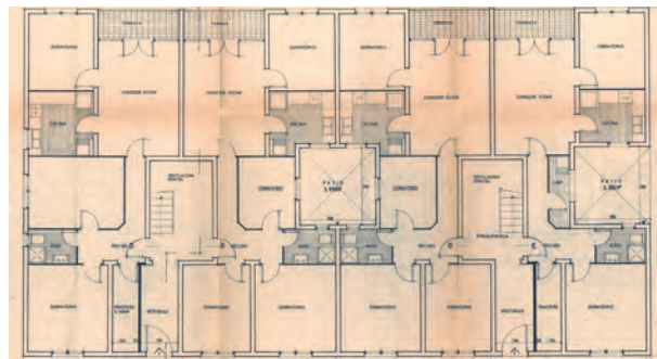
Projecte de 24 habitatges per a D. Justo Parés, 1967. (Arxiu Municipal de Manlleu)
