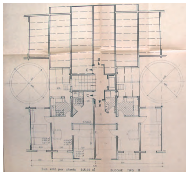
Planta tipus dels habitatges. (Arxiu Municipal de Manlleu)
